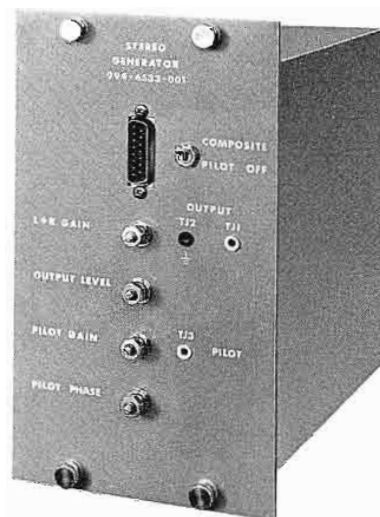
Stereo Generator Module (Optional)
